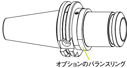
PGツールホルダ
