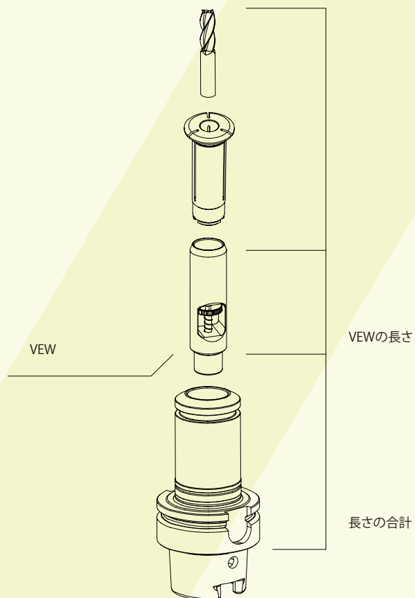
工具長プリセットツール VEW
